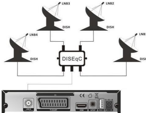
Bild 7. Anschluss an LNB-Satellitenschüssel
