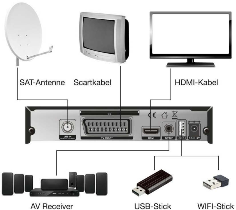
Bild 6. Anschluss an TV
